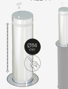
TELESCÒPICA SEMIAUTOMÀTICA amb clau Ø114 x 500m H1144
