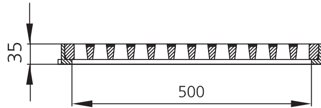
Sección AA'
