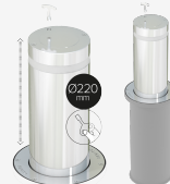
PLAZA 220 telescopico semiautomatico H2208
